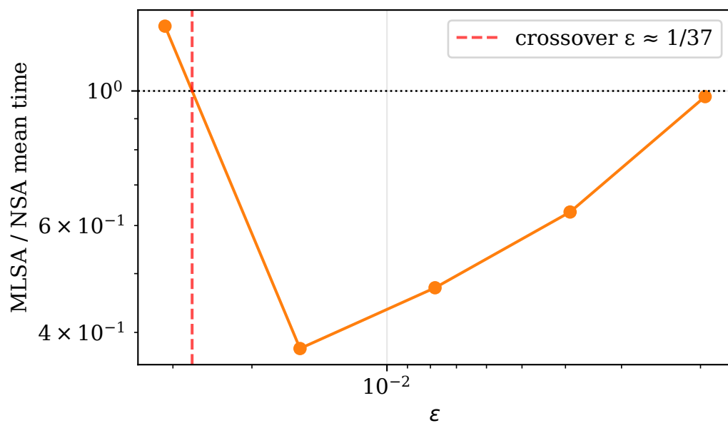
heston ES
