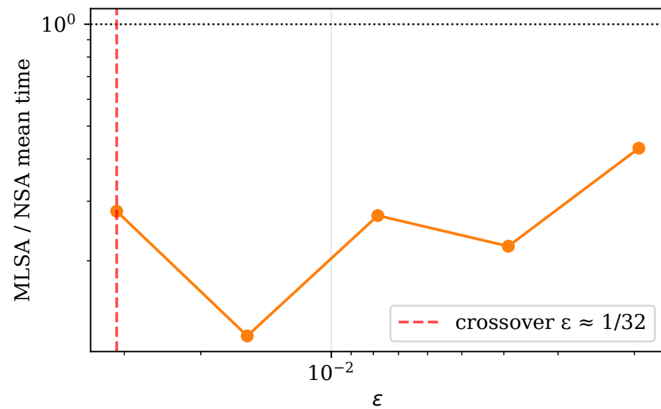
merton ES
