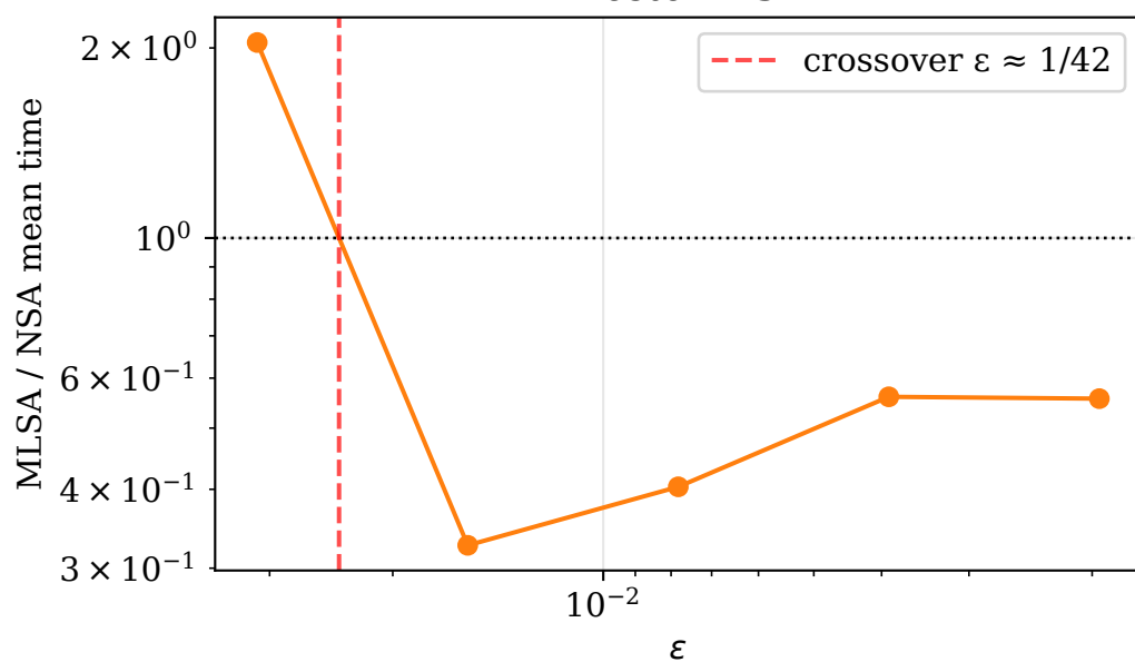
heston ES
