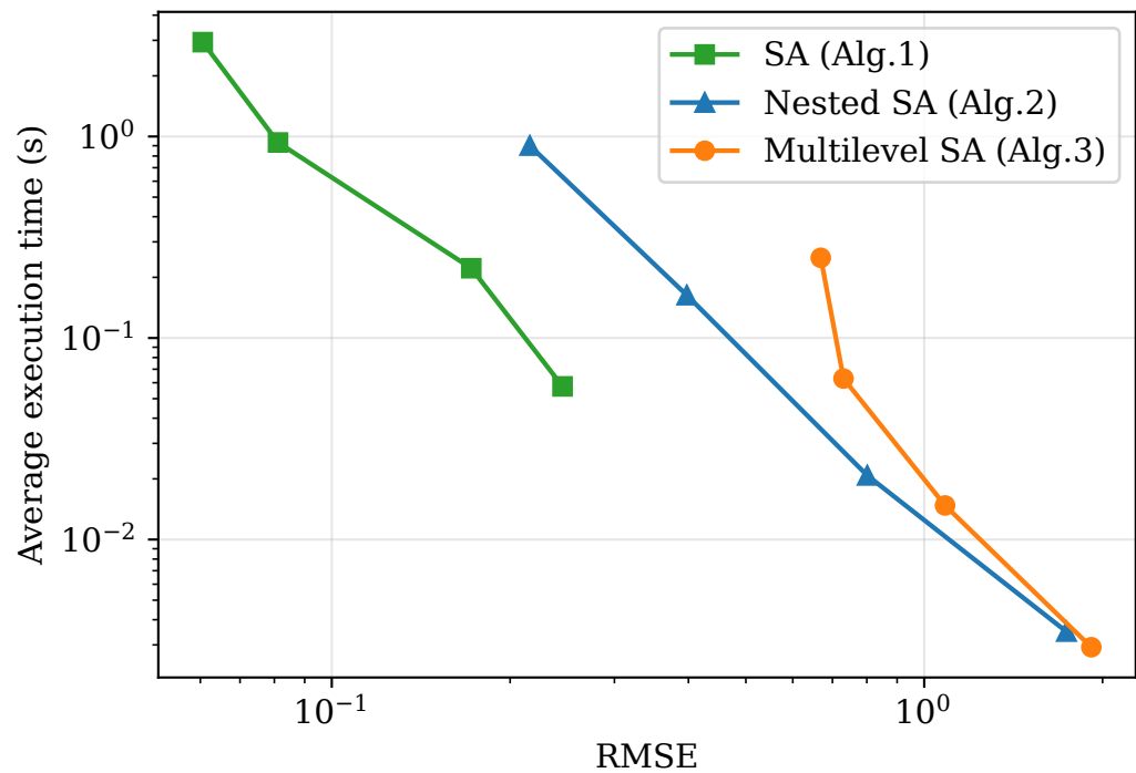
Heston ES
