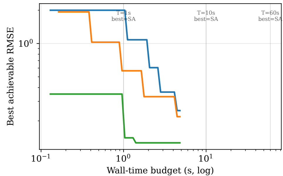
heston ES
