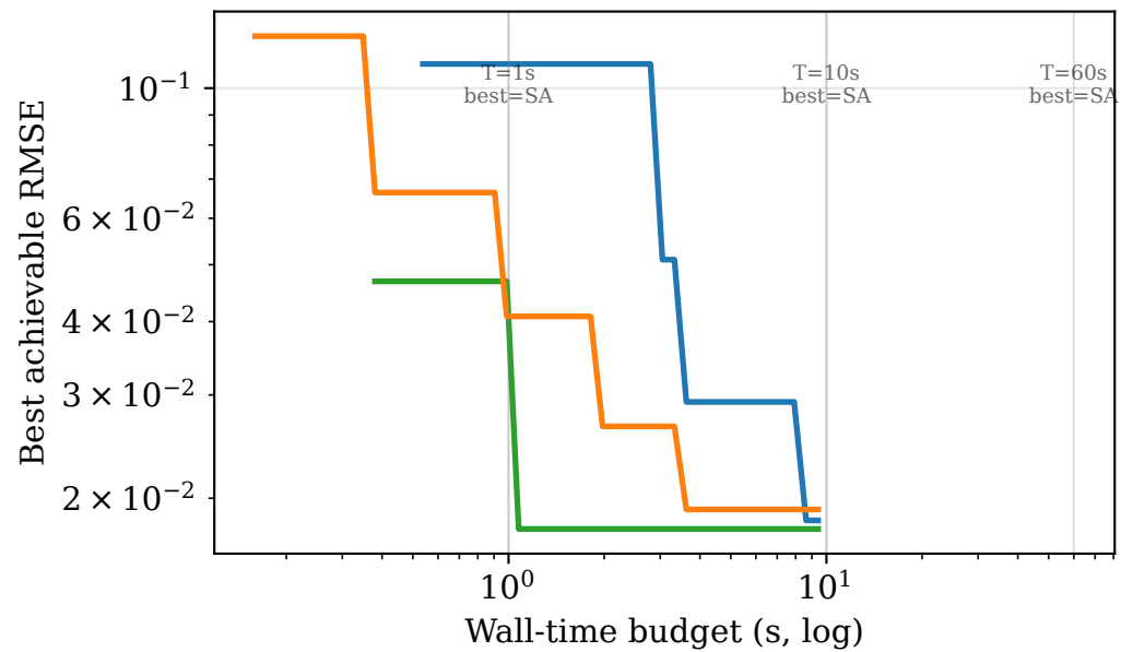
merton ES
