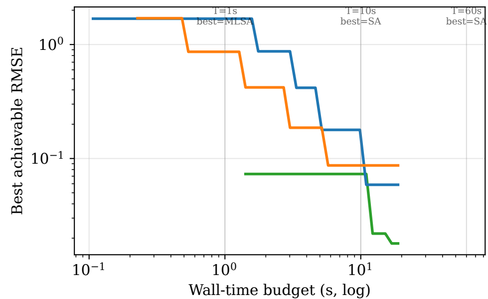
heston ES
