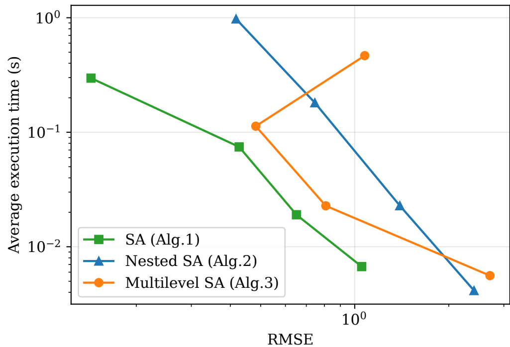
Merton ES
