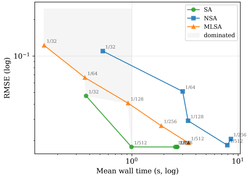
bs ES: Pareto frontier
