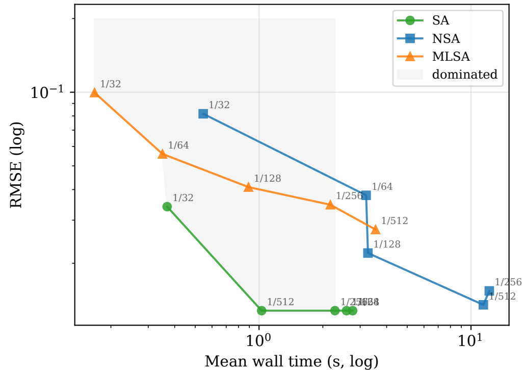
bs VaR: Pareto frontier
