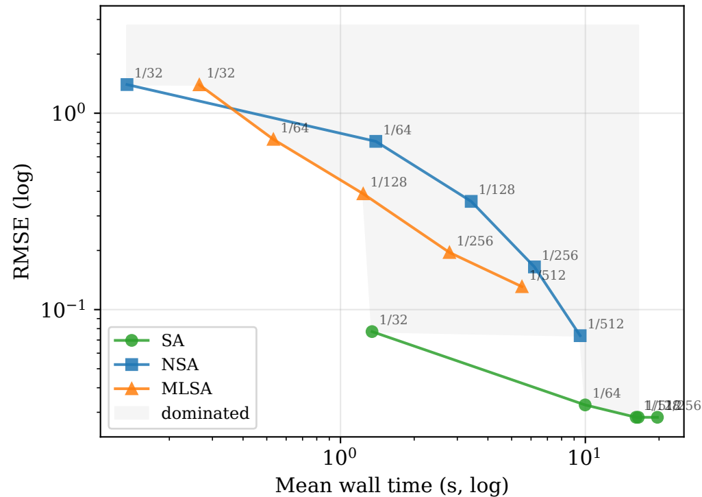
heston VaR: Pareto frontier
