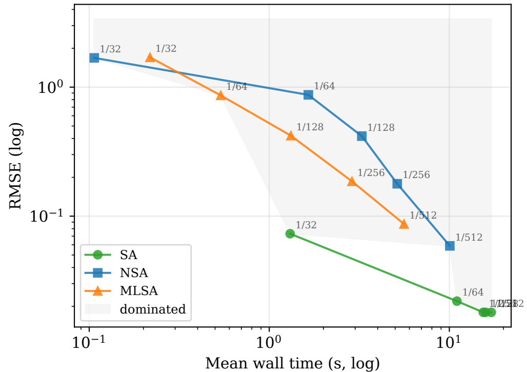
heston ES: Pareto frontier
