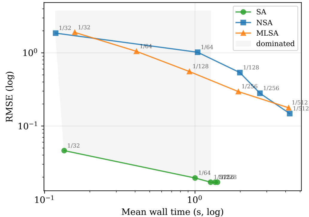
merton VaR: Pareto frontier
