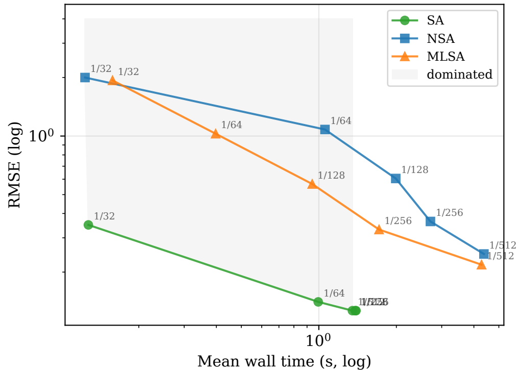
merton ES: Pareto frontier
