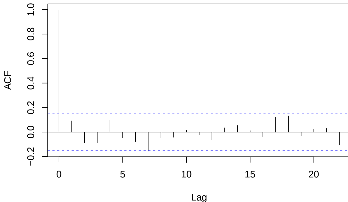
Figure 5: Gráfico da Função de Autocorrelação (ACF) dos resíduos do modelo ANOVA
