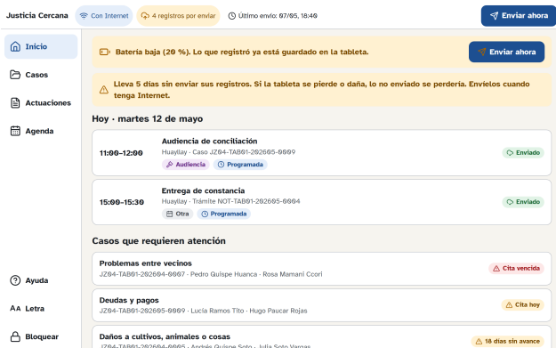
P-01. Batería baja 20 %: lo registrado ya está en la tabletta; [Enviar ahora] ( Factores humanos y dispositivo )
