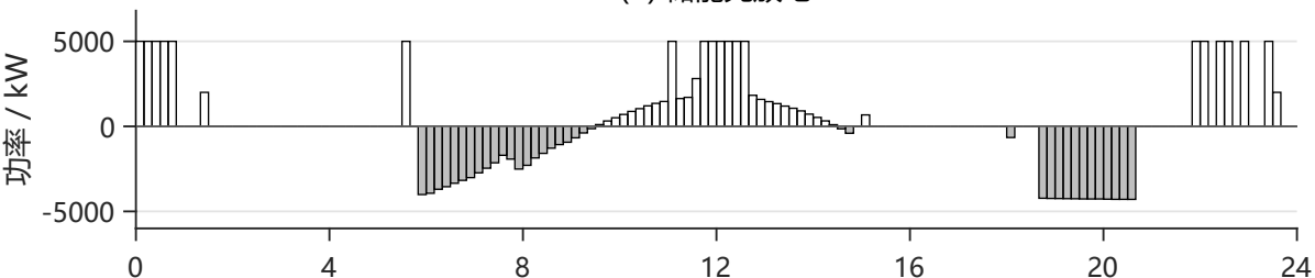
(b) 储能充放电
