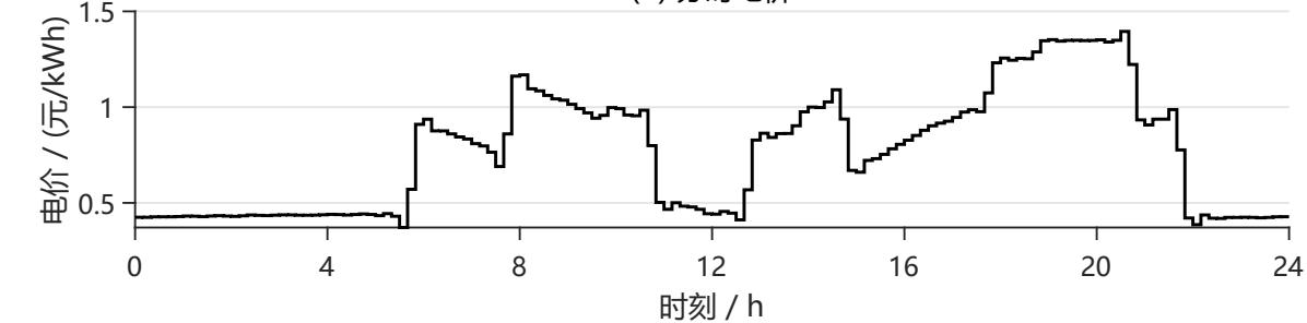
(d) 分时电价
