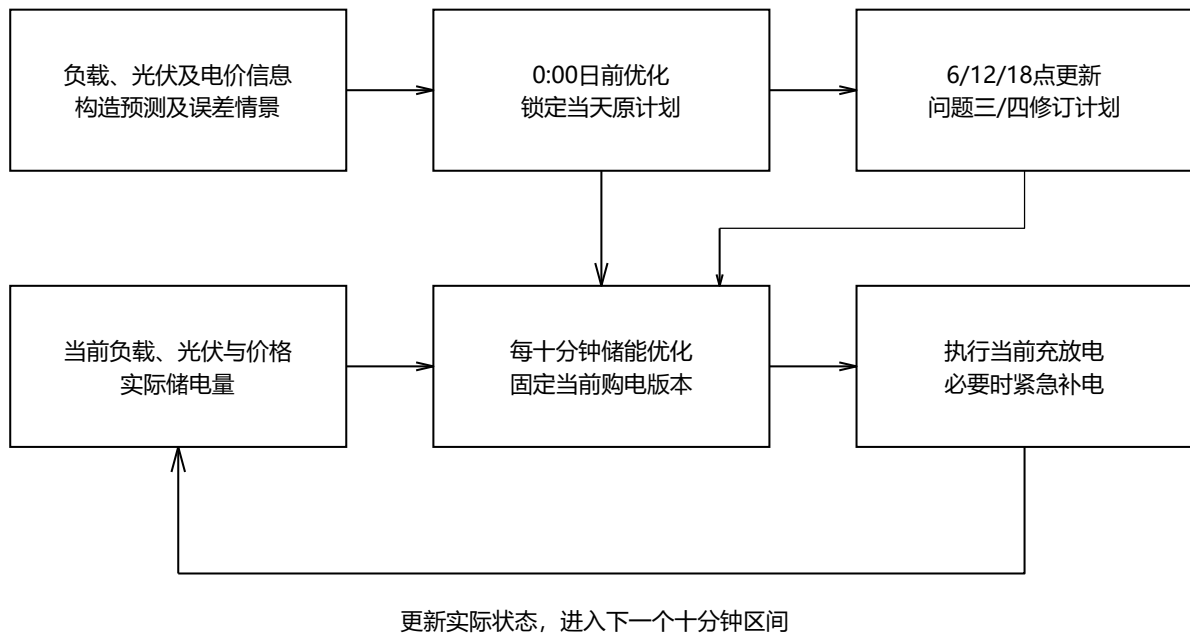
图1 日前计划、日内购电修订与实时储能执行的关系。购电修订适用于问题三及问题四的对应策略，第四问另加入电价预测与当前价格观测。
