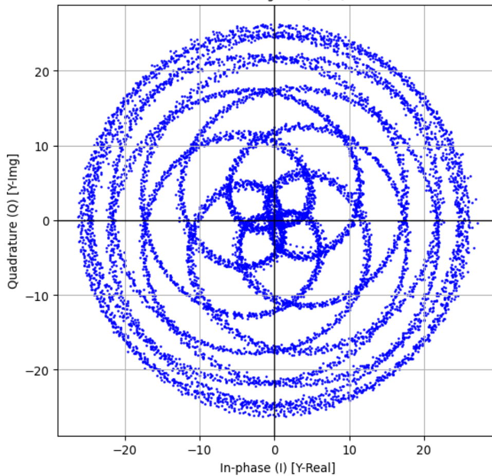
Forecast (Teste) p:1, xl:1, r:1, i:2
