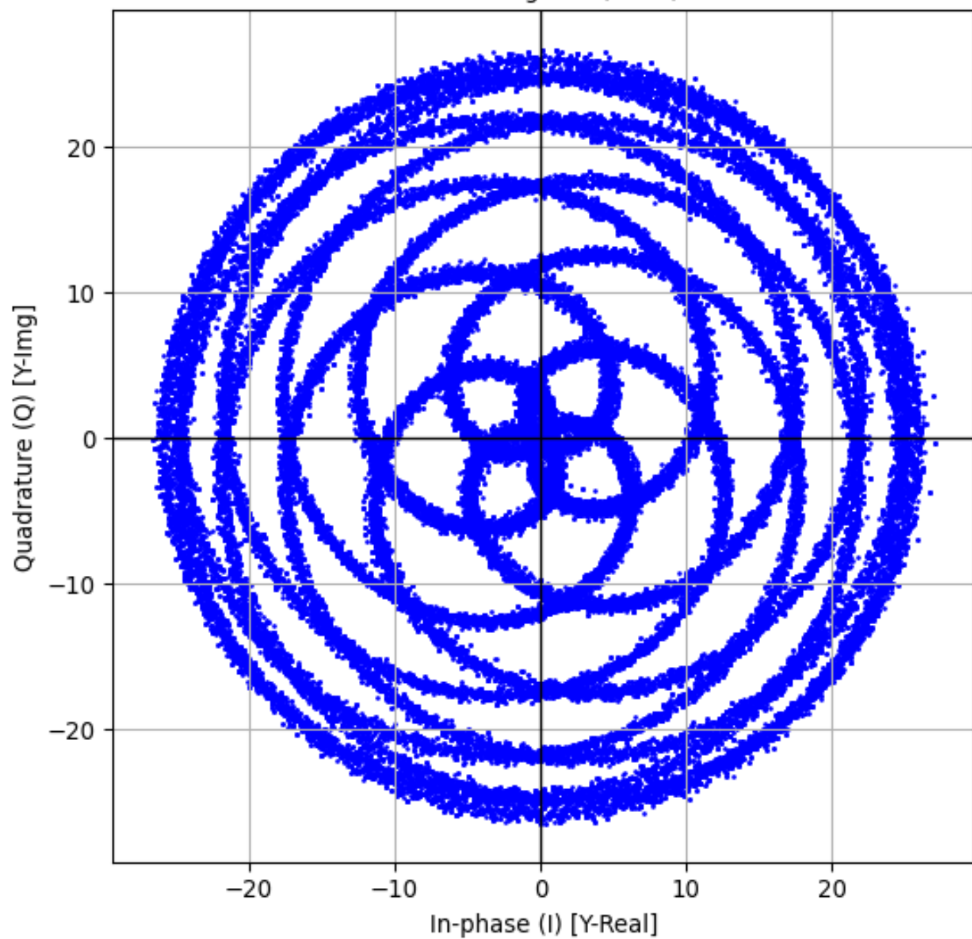
Dados Originais (Teste)
