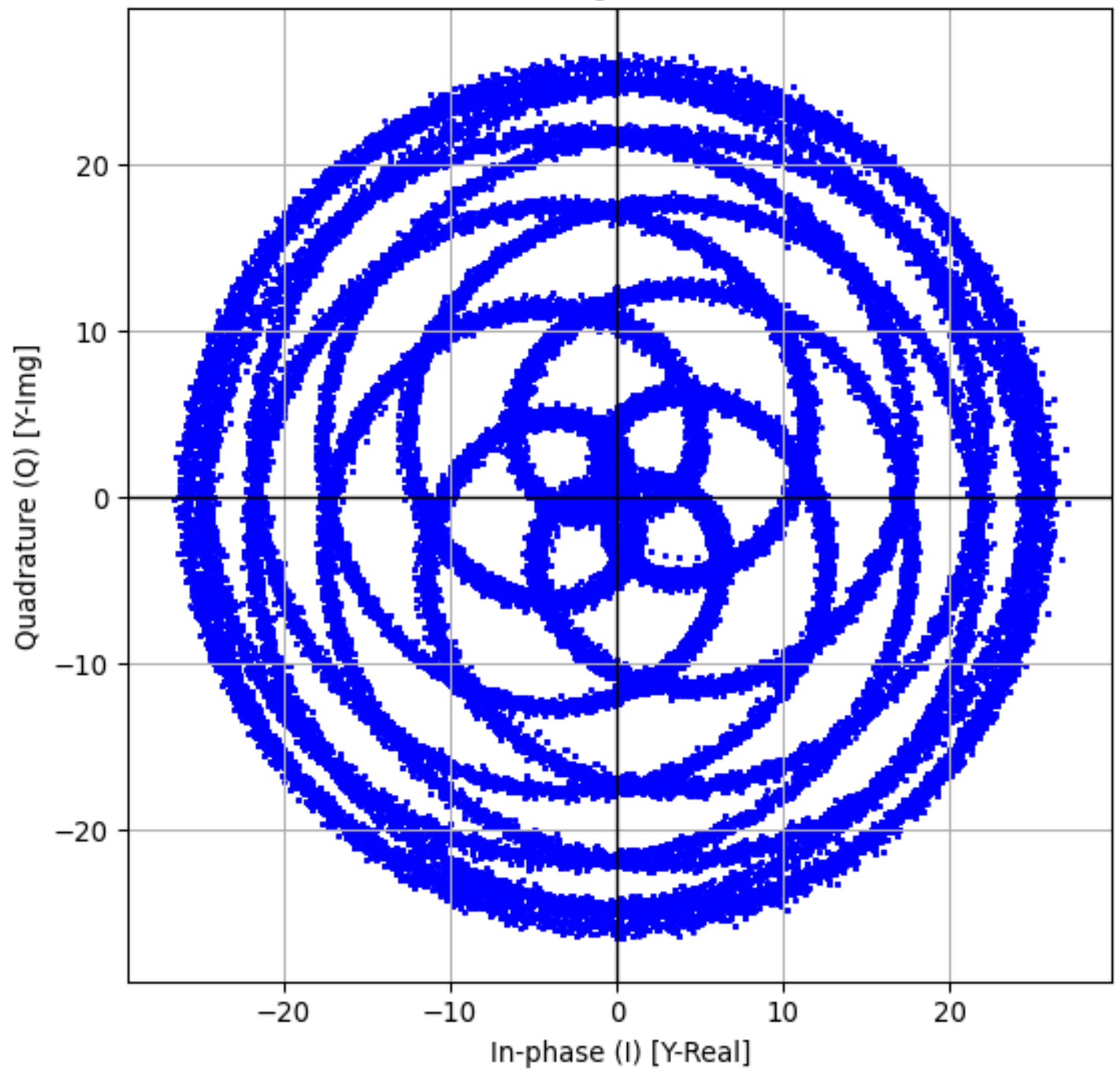
Dados Originais (Treino)
