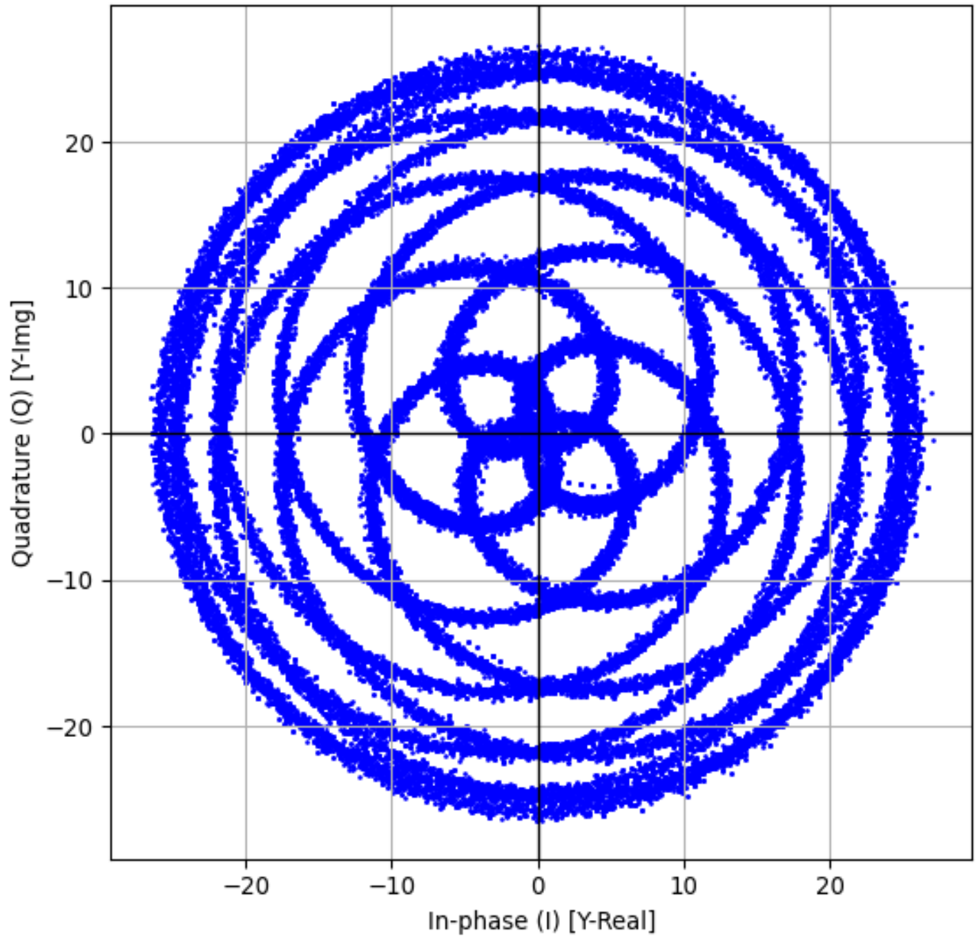
Dados Originais (Validacao)
