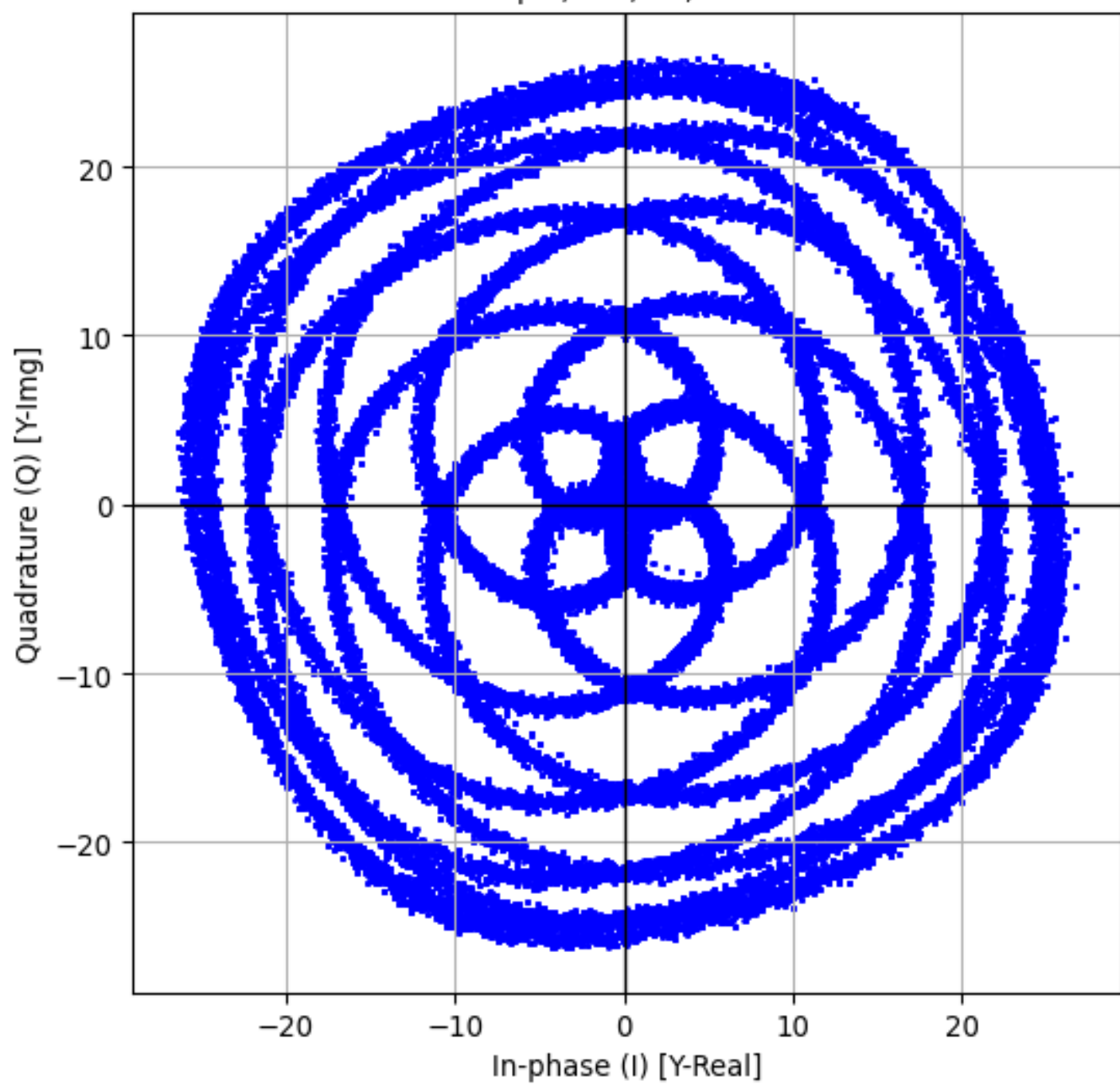
Forecast (Treino) p:2, xl:2, r:3, i:3
