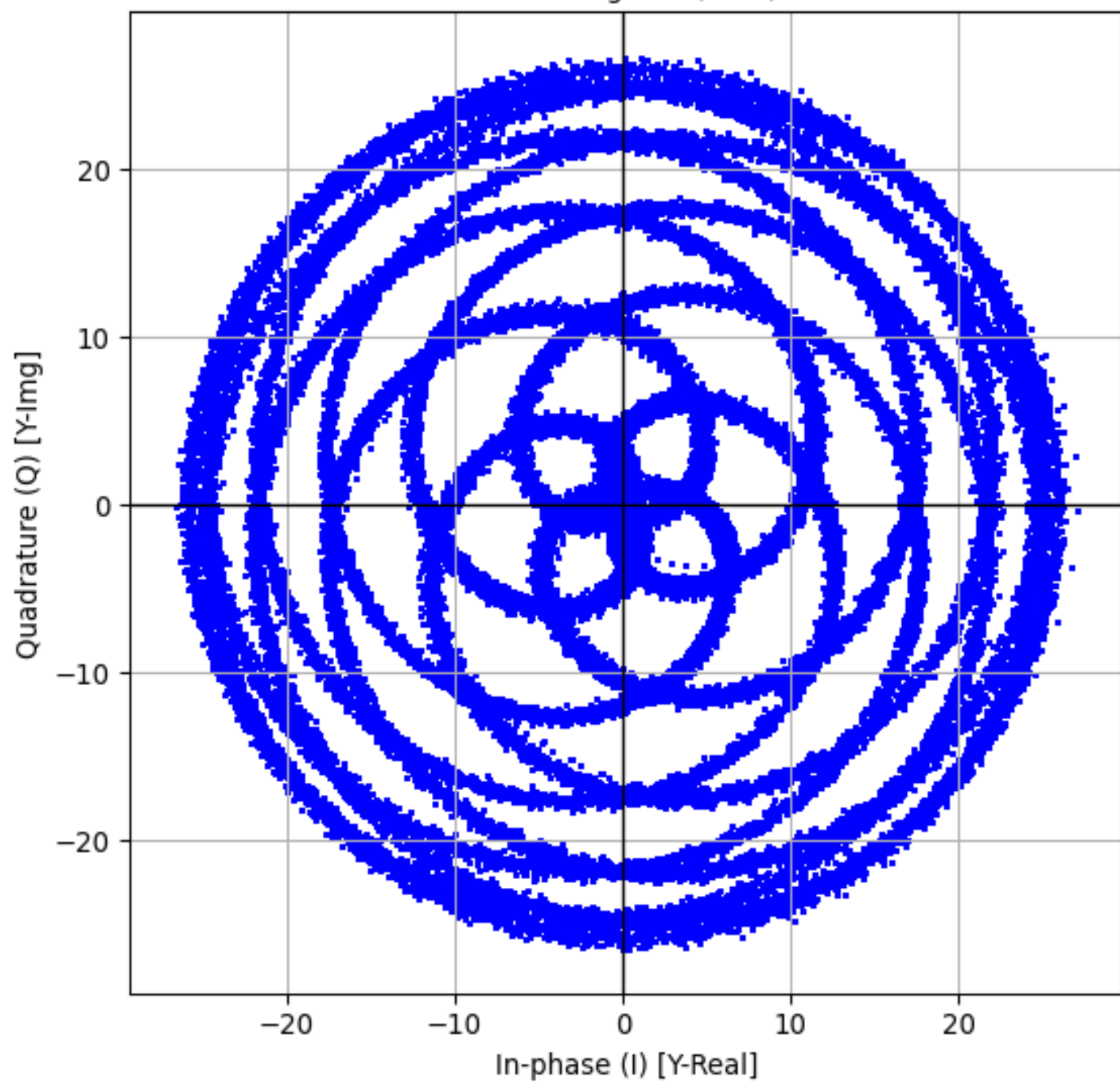
Dados Originais (Total)
