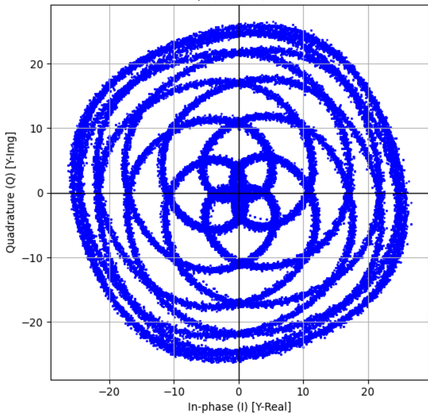
Forecast (Validacao) p:2, xl:2, r:3, i:3
