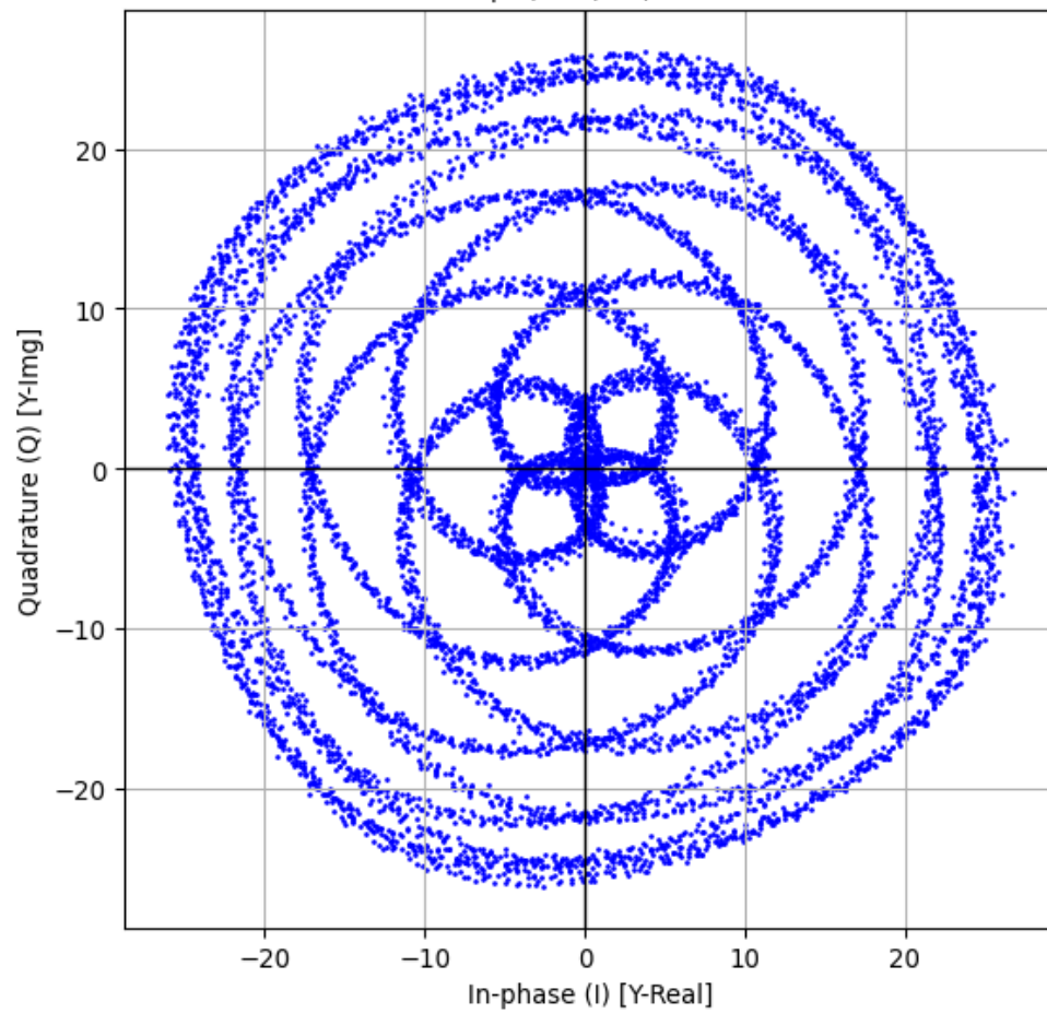
Forecast (Teste) p:2, xl:2, r:3, i:3
