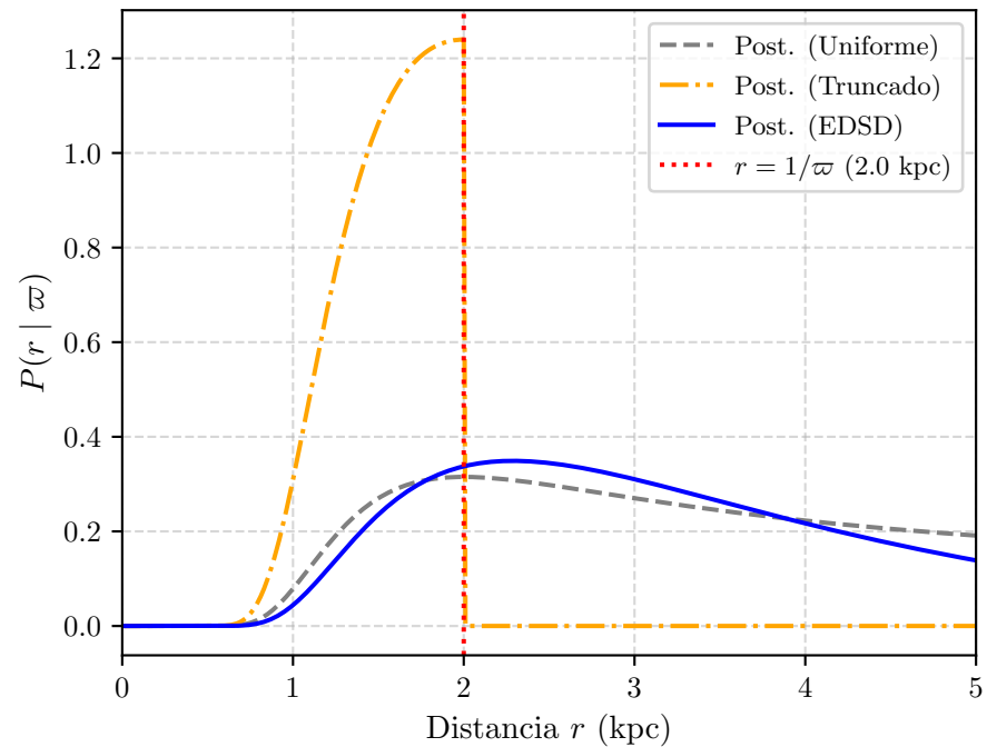
Posterior para \hat{\varpi} = 0.5 mas \sigma_{\varpi} = 0.3 mas
