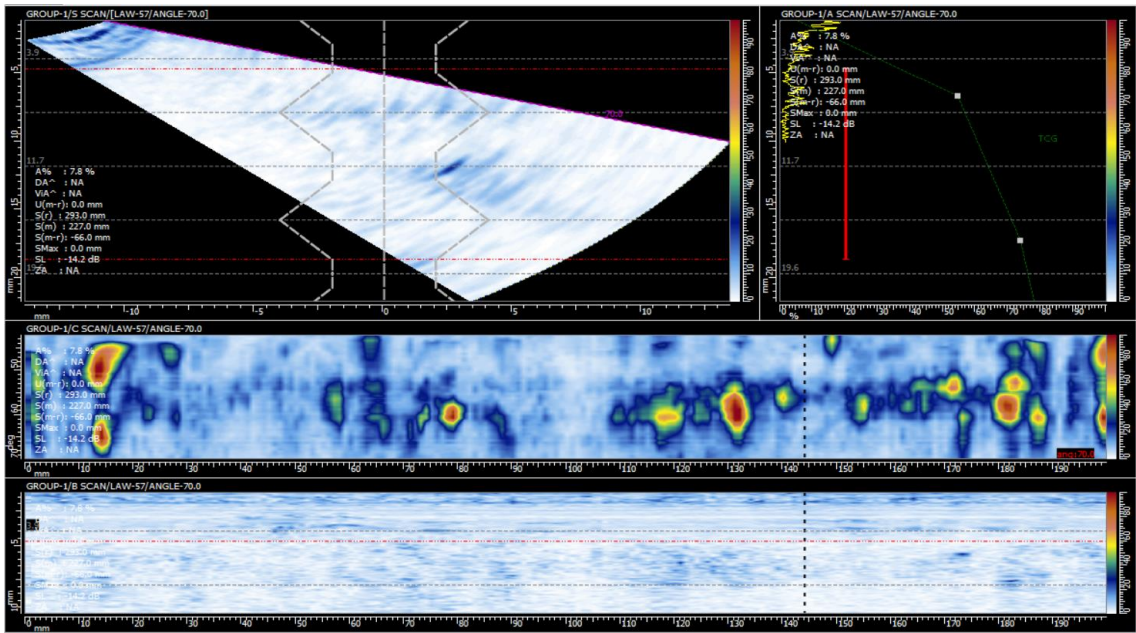
SPOOL-001 JUNTA-006
