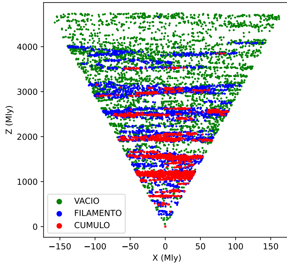
Estructuras clasificadas (VACIO verde, FILAMENTO azul, CUMULO rojo)
