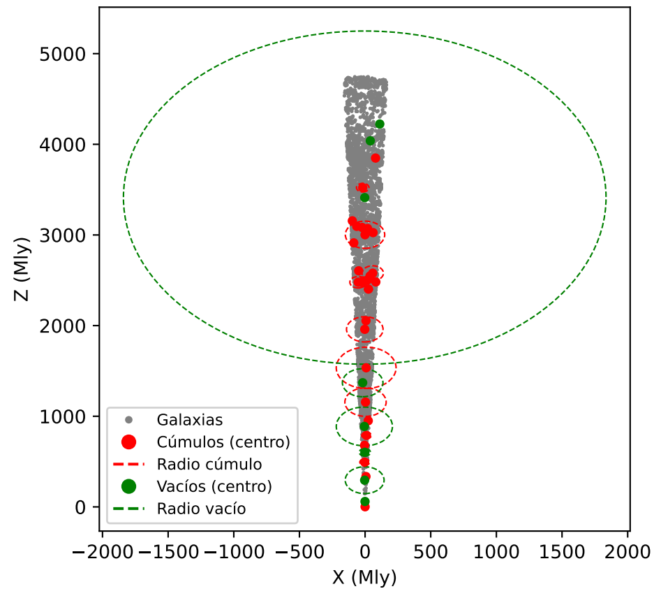
Centros y radios de cúmulos (rojo) y vacíos (verde)
