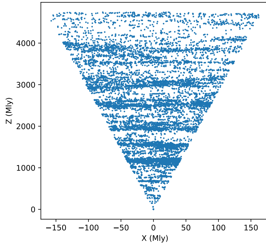
Distribución de galaxias (proyecciones 2D)
