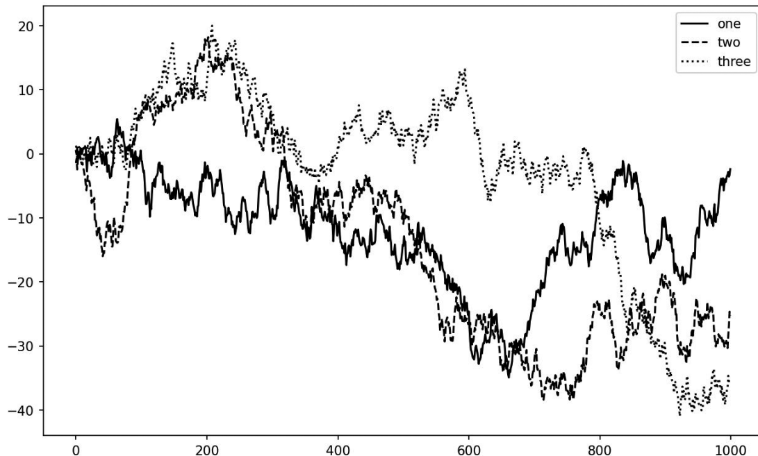
Figura 9.10. Sencillo gráfico con tres línea y leyenda.
