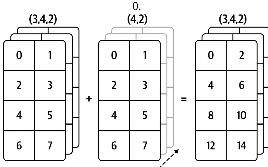
Figura A.6. Difusión a lo largo del eje 0 de un array tridimensional.
