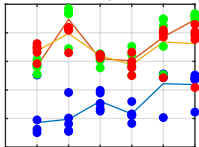
TCA cycle
