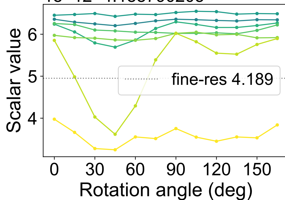
(d) w300 (Euler char.) 1e-12+4.188790205
