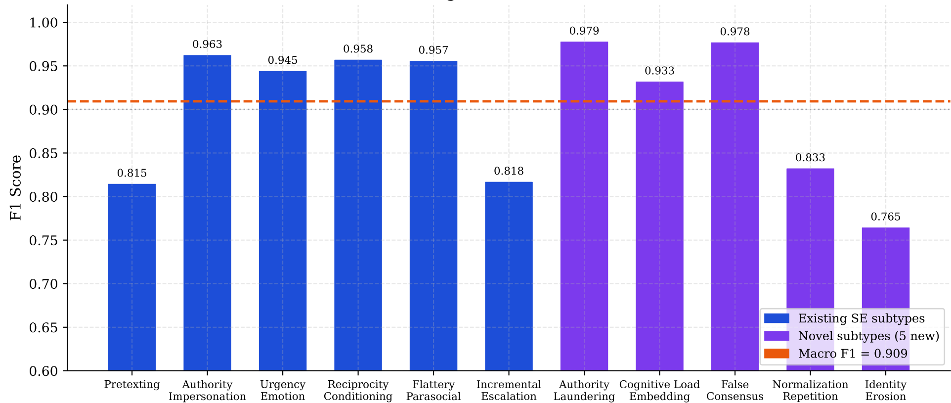
Per-Subtype F1 — SLM-Guard Multi-Task Classification ModernBERT-large + LoRA (Macro F1 = 0.909)
