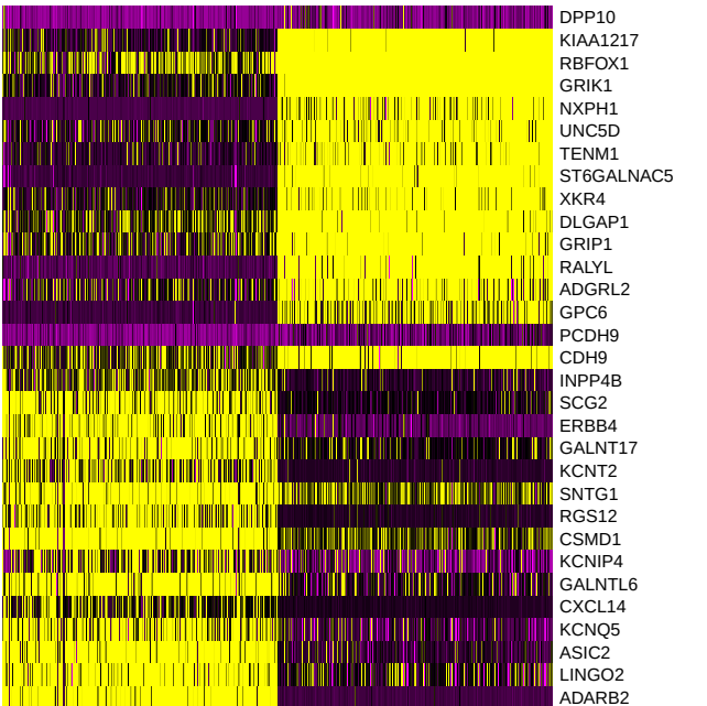
PC_7
