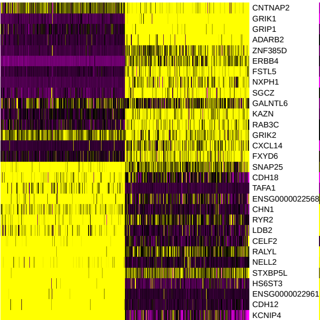
PC_5
