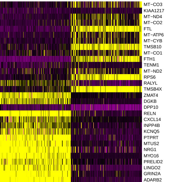
PC_9
