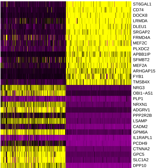
PC_4
