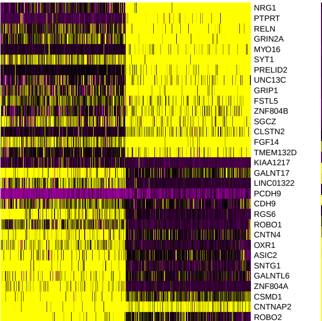
PC_8
