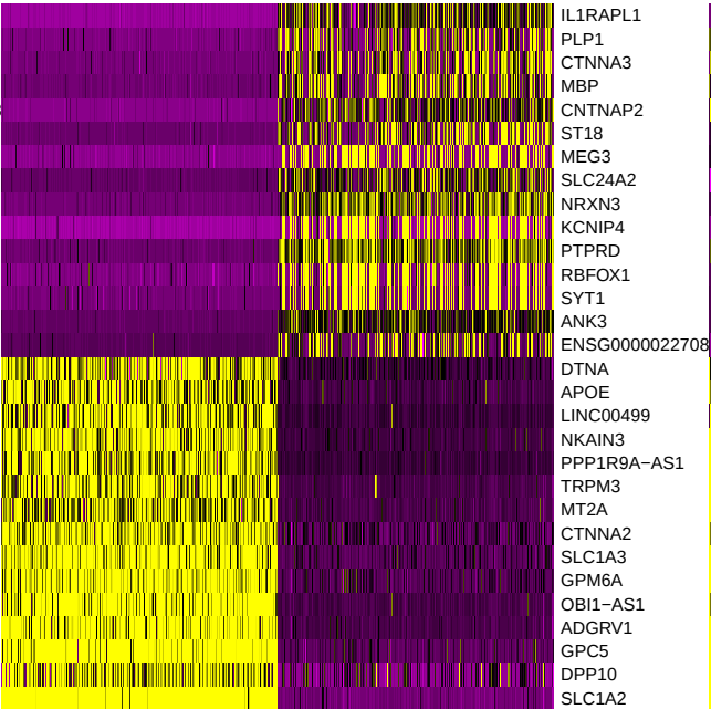
PC_2
