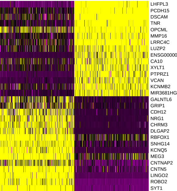
PC_3
