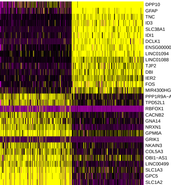
PC_6
