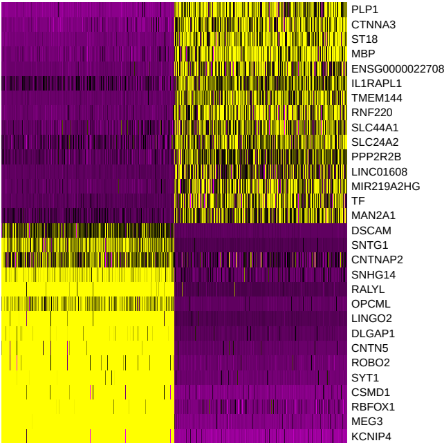
PC_1
