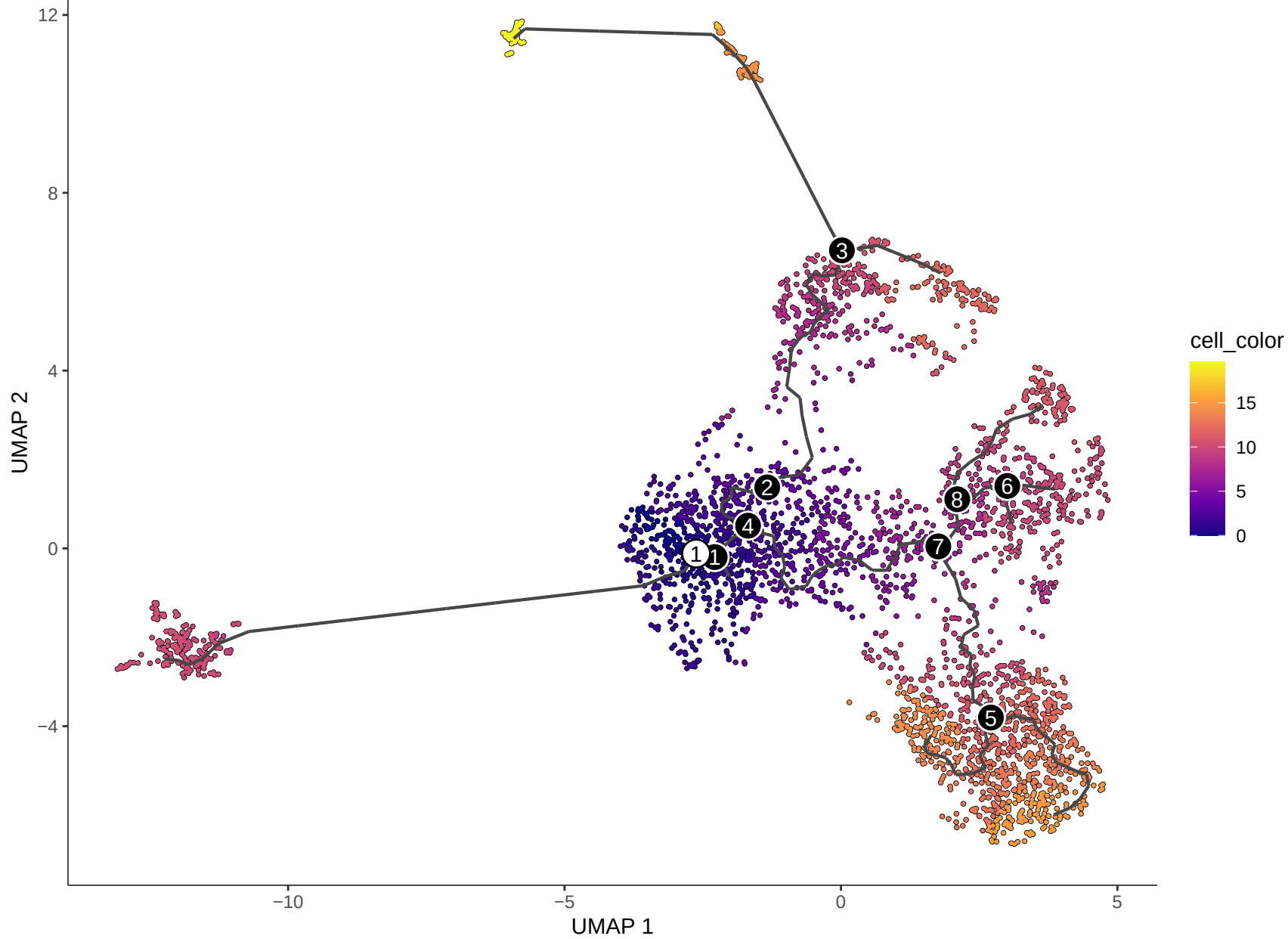
MicrogliaActivation — pseudotime
