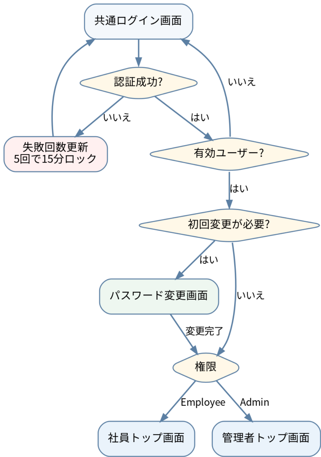
図 9-1 認証処理フロー
