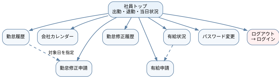
図 6-2 社員画面遷移
