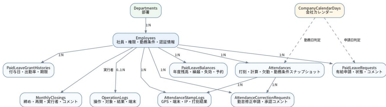
図 10-1 主要テーブル関連概要
