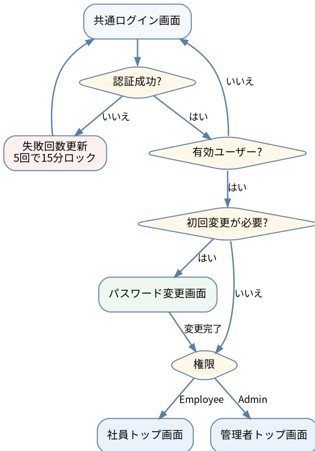
図 6-1 認証・初回パスワード変更・権限別遷移
