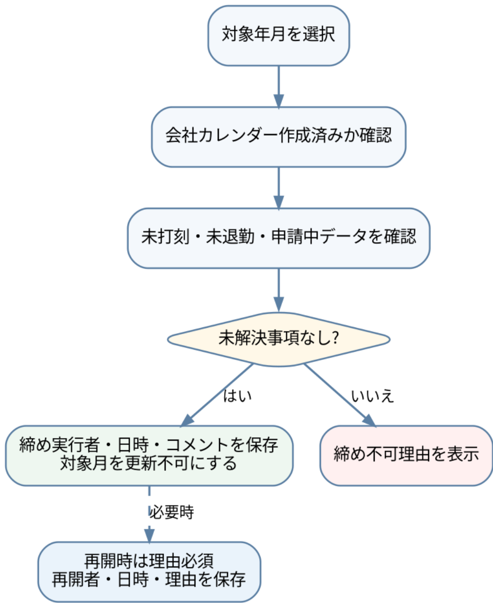
図 9-5 月次締め・再開フロー
