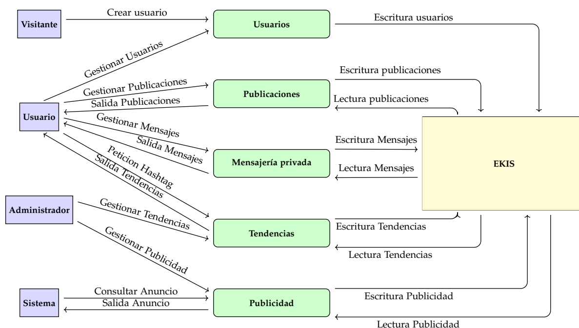
Figura 6: DFDo — Sistema EKIS
