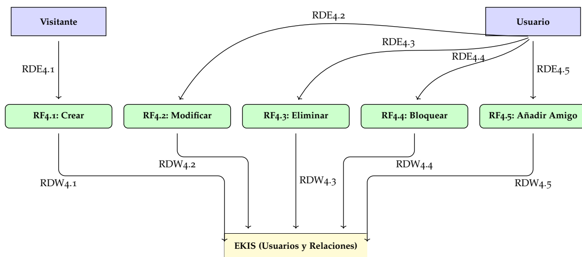
Figura 4: DFD1 - Subsistema de Usuarios
