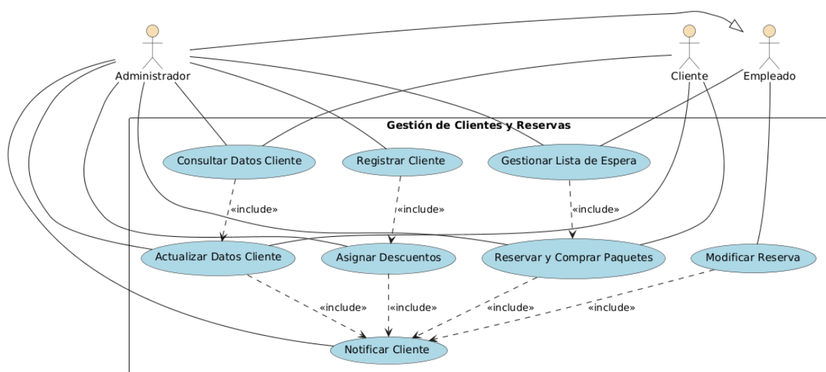
Figura 1: Diagrama de casos de uso correspondiente a la gestión de clientes y reservas.
