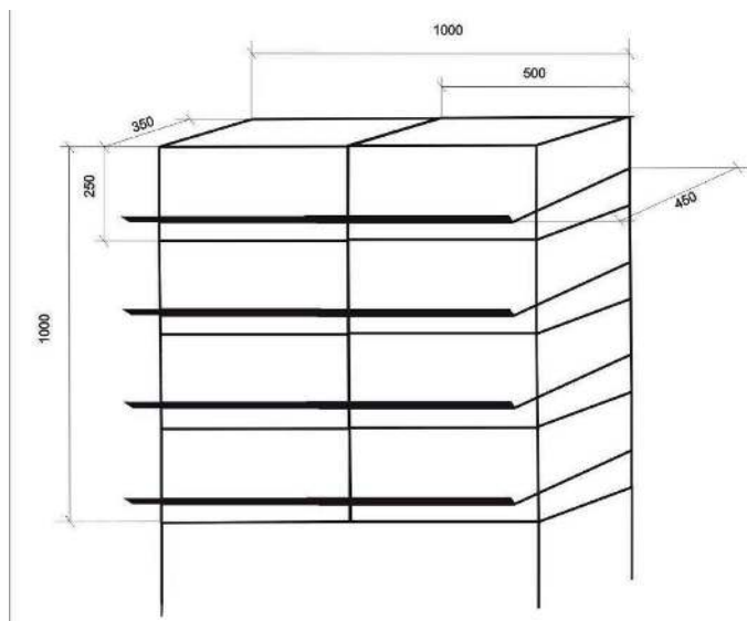
Беданаларни боқиш учун мўлжалланган универсал каток – брудер (кўп секцияли, 4 ярусли)
