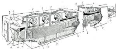
13 - расм. Тунелли кучли музлатгич жиҳозлари
