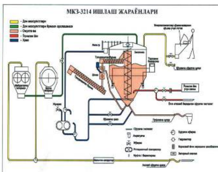
17-расм. Омихта ем ишлаб чиқарувчи мобил (МКЗ) заводи
