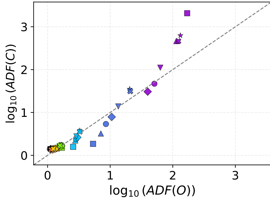
(a) Densidad constante
