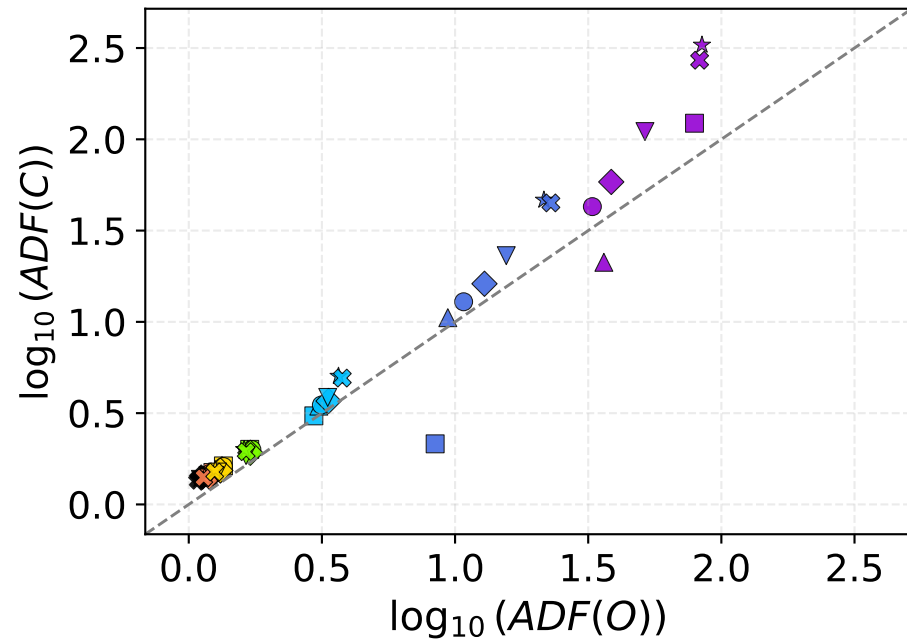
(c) Modelos ópticamente delgados
