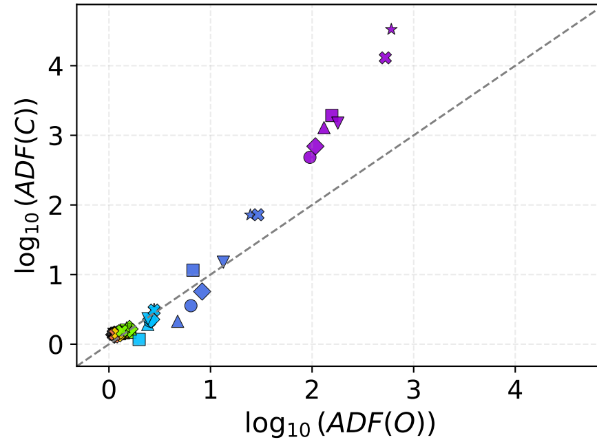
(b) Presión constante
