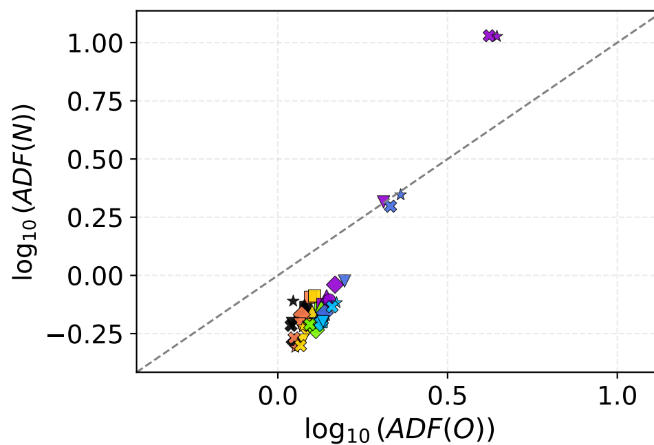
(d) Modelos con polvo proporcional al enriquecimiento
