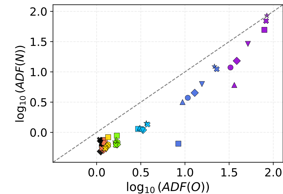
(c) Modelos ópticamente delgados
