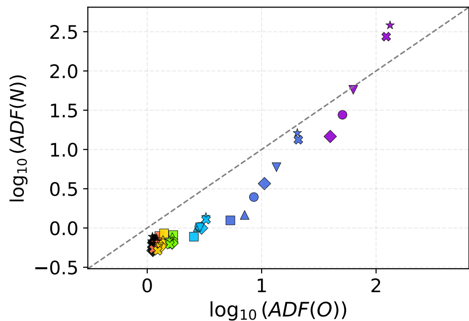
(a) Densidad constante
