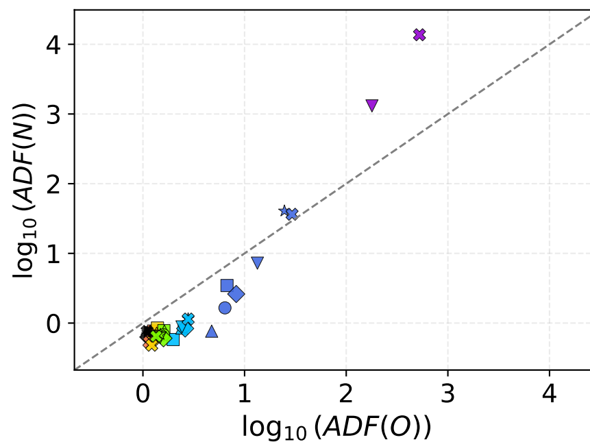
(b) Presión constante
