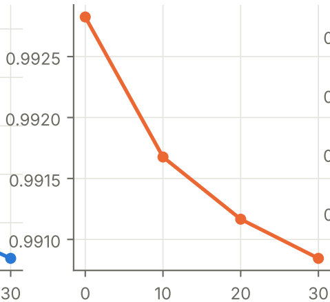
AUPRC
