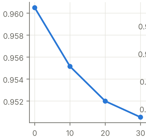
ROC-AUC
