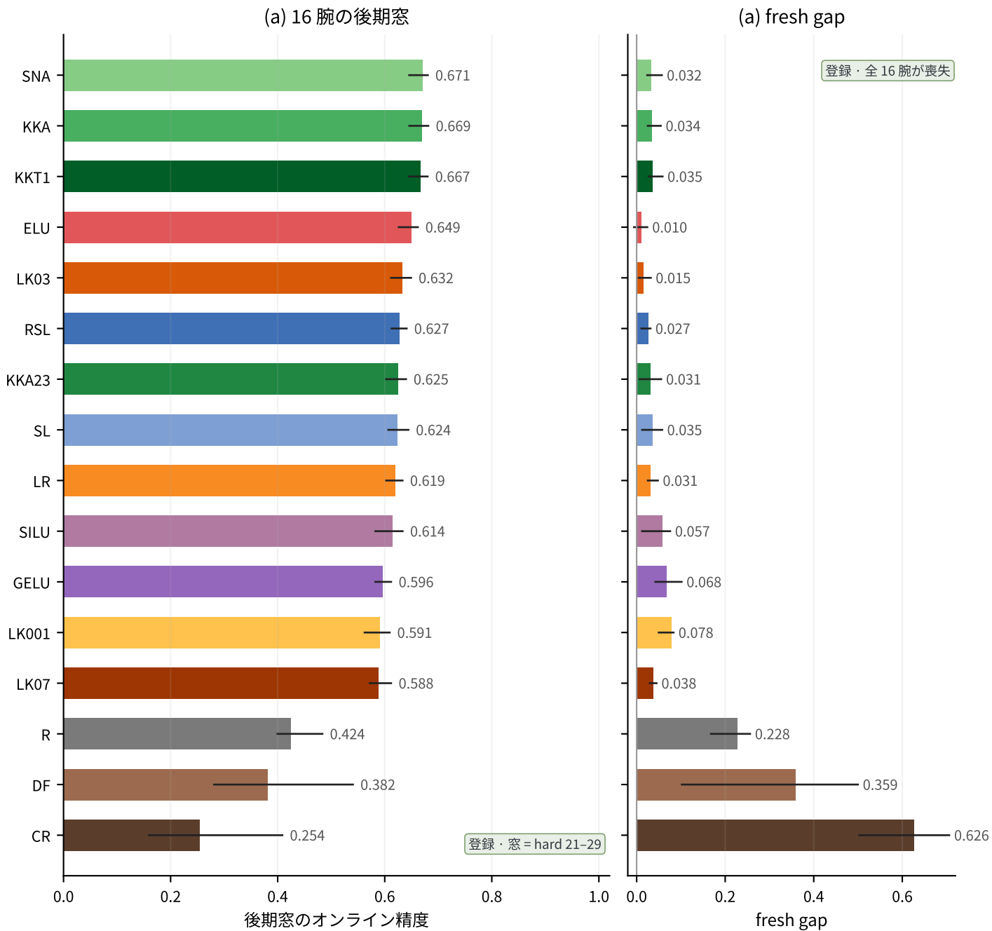
図 10 実ラベルの箱 — 5+1 CIFAR / MLP ・ 30 課題 ・ 10 seed
