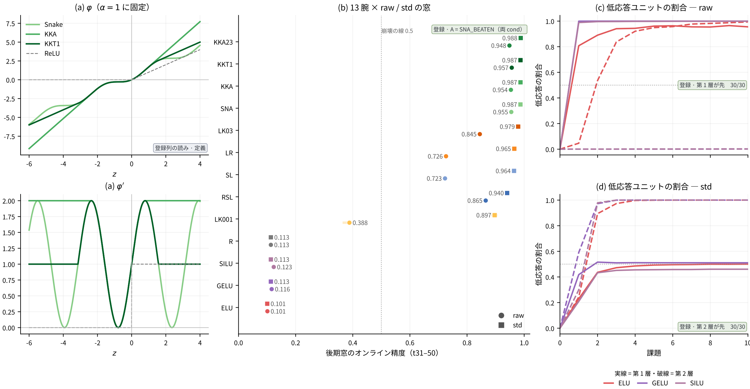
図 7 活性化 — RL-CIFAR / MLP・50 課題・10 seed
