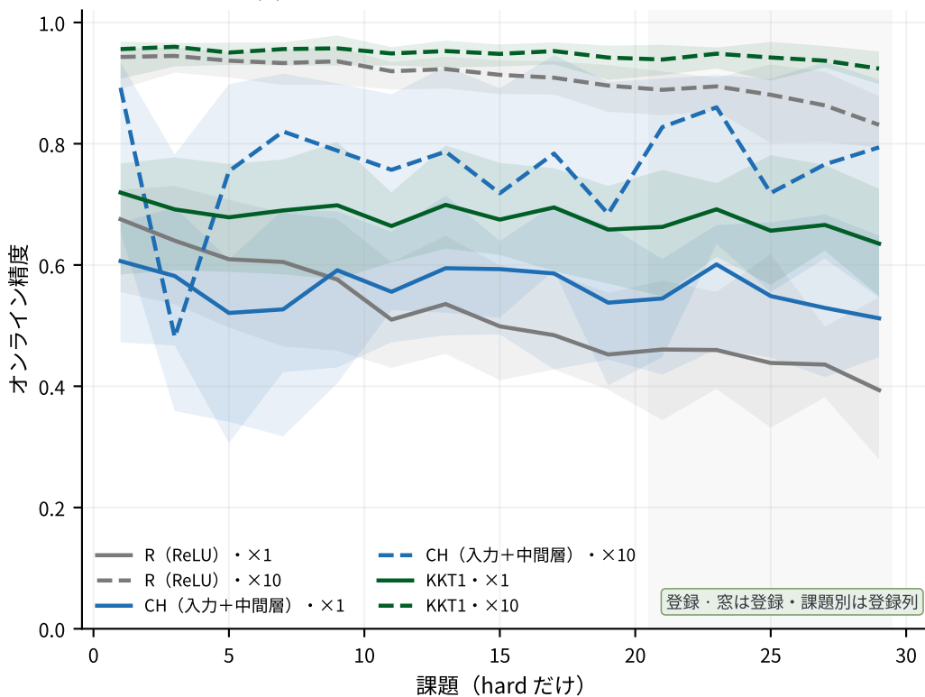
(a) 課題別 online: ×1 (実線) 対 ×10 (破線)
