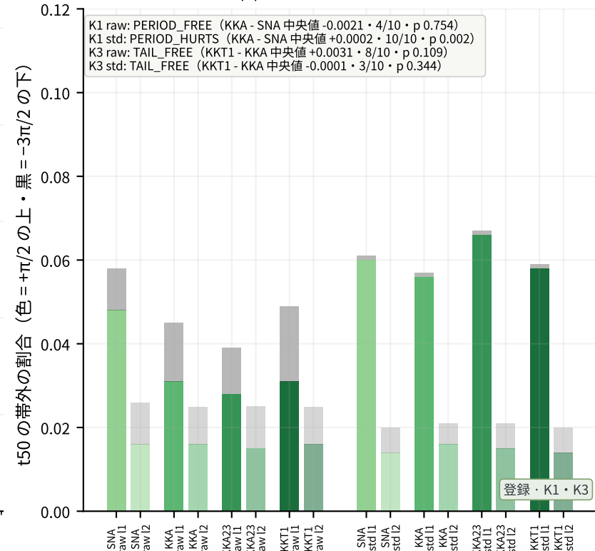
(c) t50 の内訳と K1 • K3
