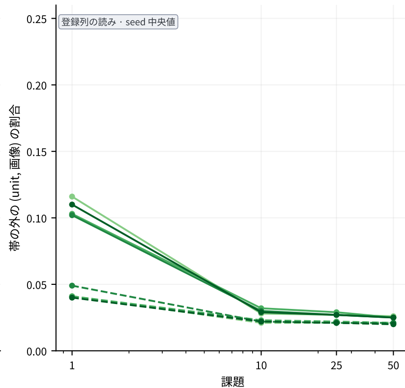
(b) 第2層: 帯 [-3\pi/2, +\pi/2] の外
