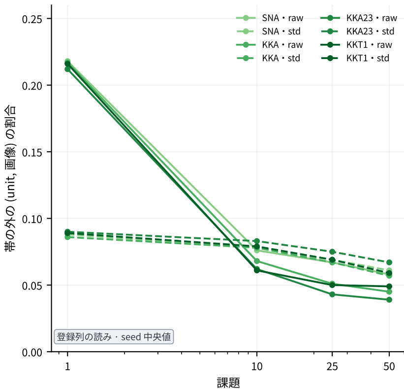
(a) 第1層: 帯 [-3\pi/2, +\pi/2] の外
