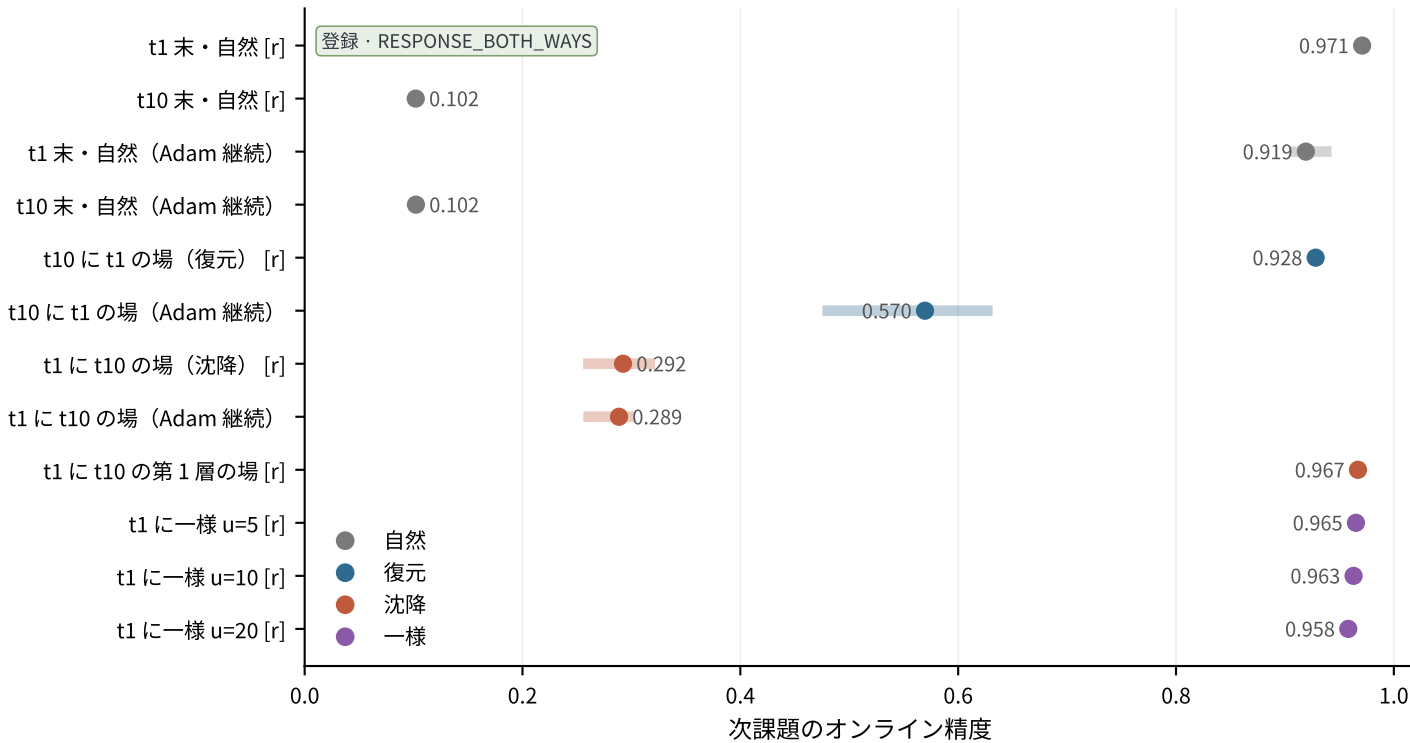
(a) 次課題の学習 ([r]: Adam 履歴初期化)
