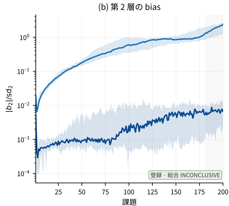
図3 bias 経路 — CH と CHB を 200 課題まで ・ 10 seed
