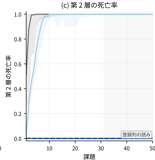
図2 中心化の扉 — RL-CIFAR / MLP・50 課題・10 seed
