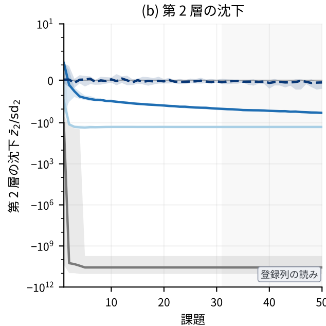
図2 中心化の扉 — RL-CIFAR / MLP・50 課題・10 seed
