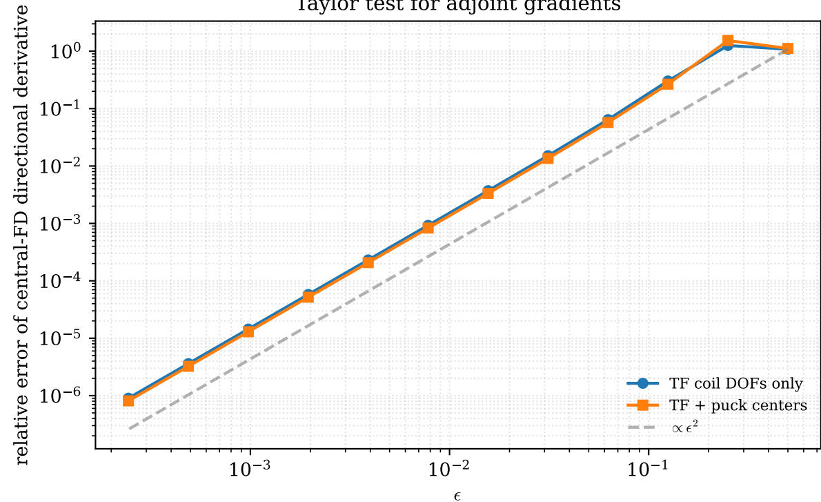
Taylor test for adjoint gradients
