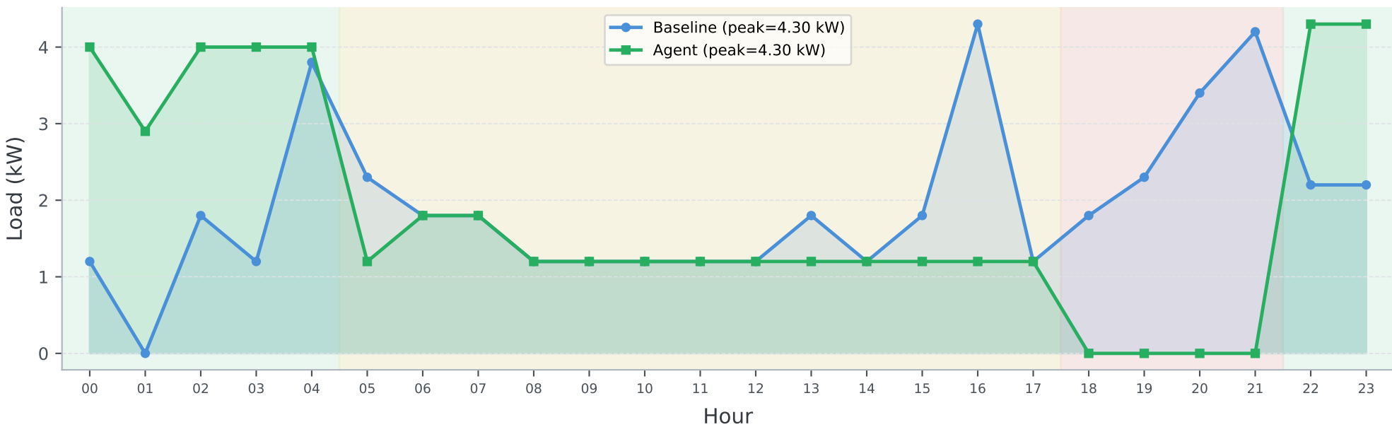
(d) Hourly Load Profile (kW)
