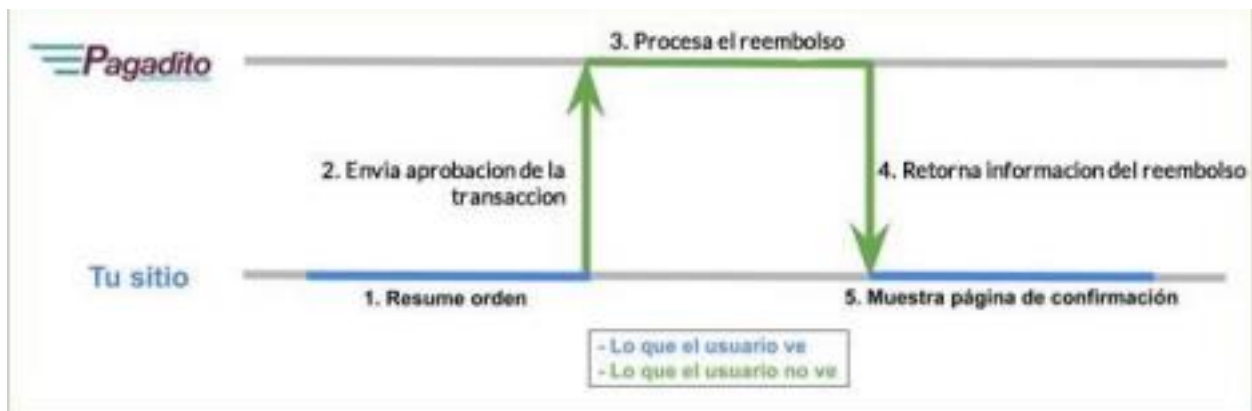
Proceso de Reembolso con Pagadito
