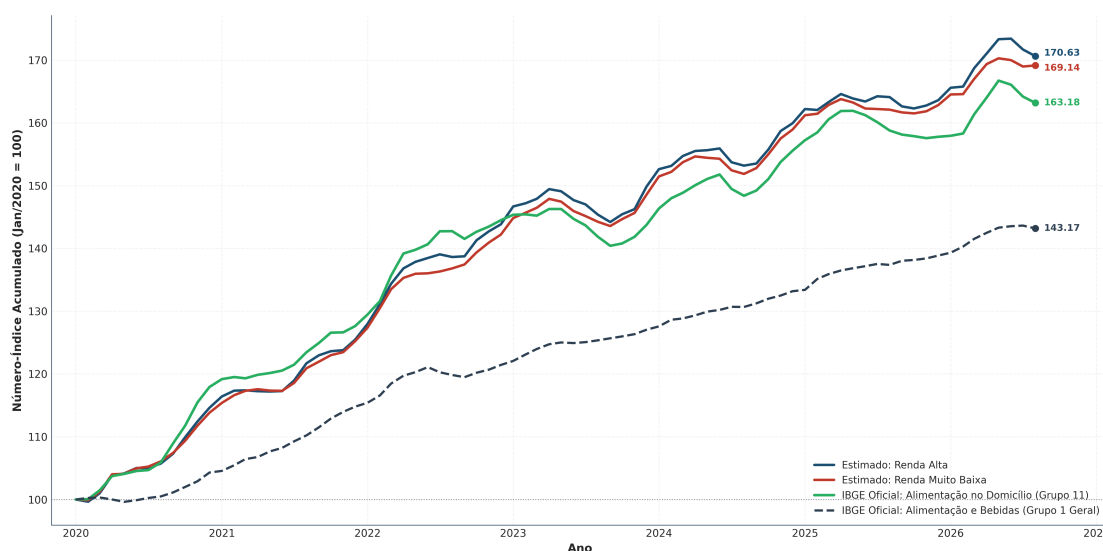
Figura 2: Validação Gráfica de Aderência: Séries Extremas Estimadas versus Séries Oficiais do IPCA/IBGE (Base: Jan/2020 = 100 | Dados até Agosto de 2026).
