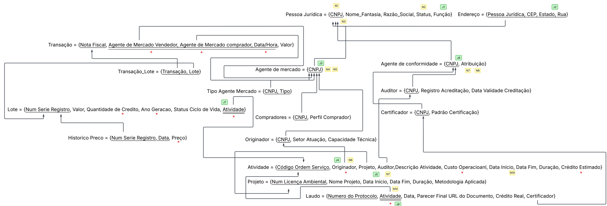
Figura 2: Diagrama do Modelo Relacional do projeto CarbonTrack.
