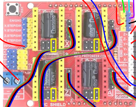
CNC Arduino shield (Place onto Arduino Uno)
