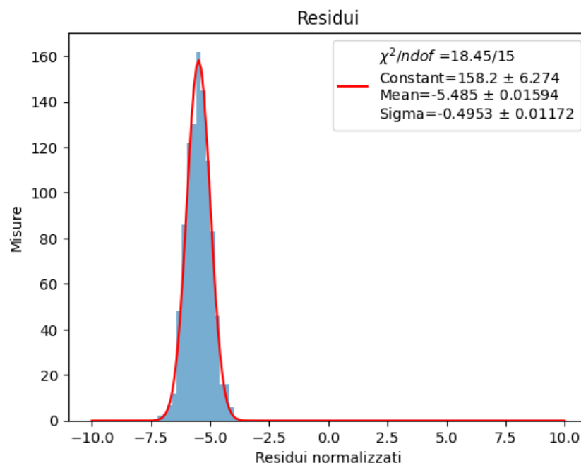
Figura 1.1: Fit di un set di dati generati casualmente secondo una distribuzione Normale ( \mu = -5.5, \sigma = 0.5 ). La curva rossa rappresenta la funzione di fit ottimizzata tramite minimizzazione del \chi^2 . Il box in alto a destra, generato da iminuit , riporta i parametri estratti e i relativi errori.
