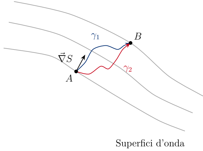
Figura 1.3: Propagazione tra superfici d'onda e percorsi alternativi.
