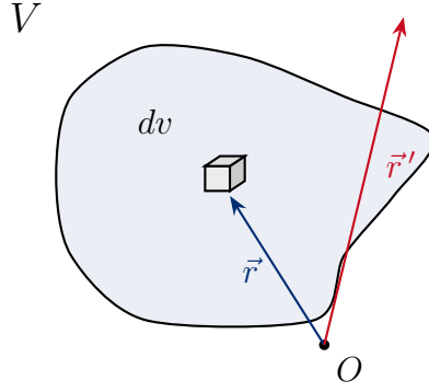
Figura 1.4: Elemento di volume dv all'interno del volume V .
