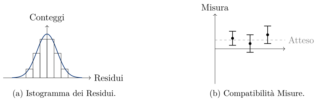
Figura 1.6: Diagnostica statistica post-fit.
