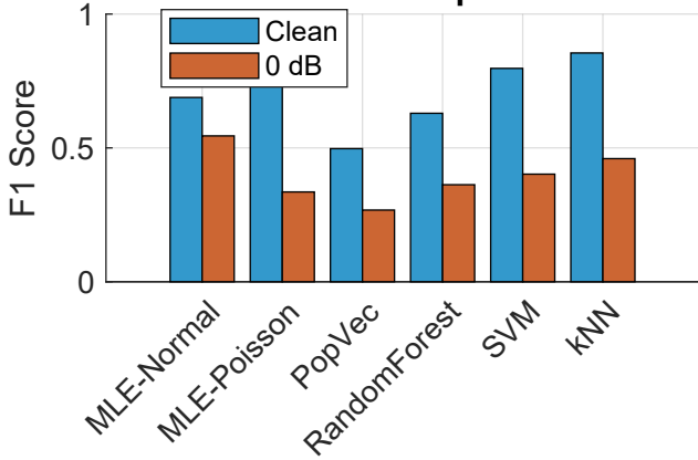
F1 Score Comparison
