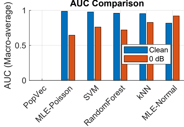
AUC Comparison
