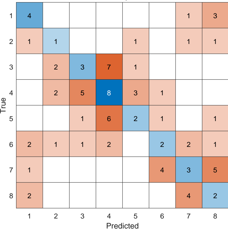
Confusion: PopVec @ 0 dB
