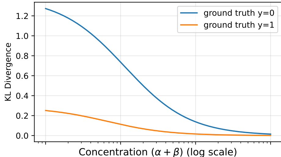
KL Divergence Fixed \mu=0.75
