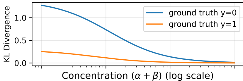
KL Divergence Fixed \mu=0.75
